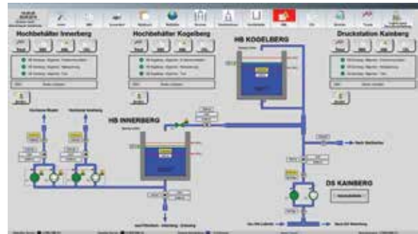
Abbildung 2: Der Detailgrad der Stationsübersicht – einzelne Teilanlagen oder größere zusammenhängende Anlagenteile – ist frei wählbar.
